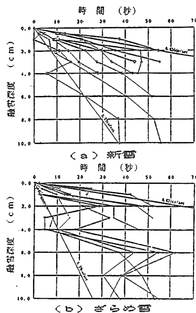
図-1 融雪深度と時間
