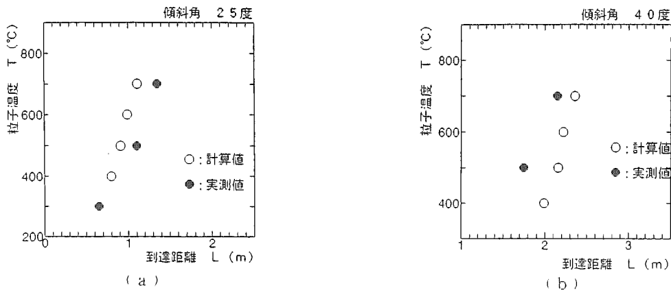
図-8 計算値と実測値
