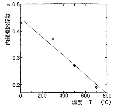
図-7 砂温度と内部摩擦係数
