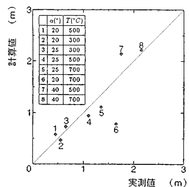
図-9 到達距離の整合性
