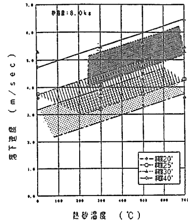
図-4 砂温度と落下速度
