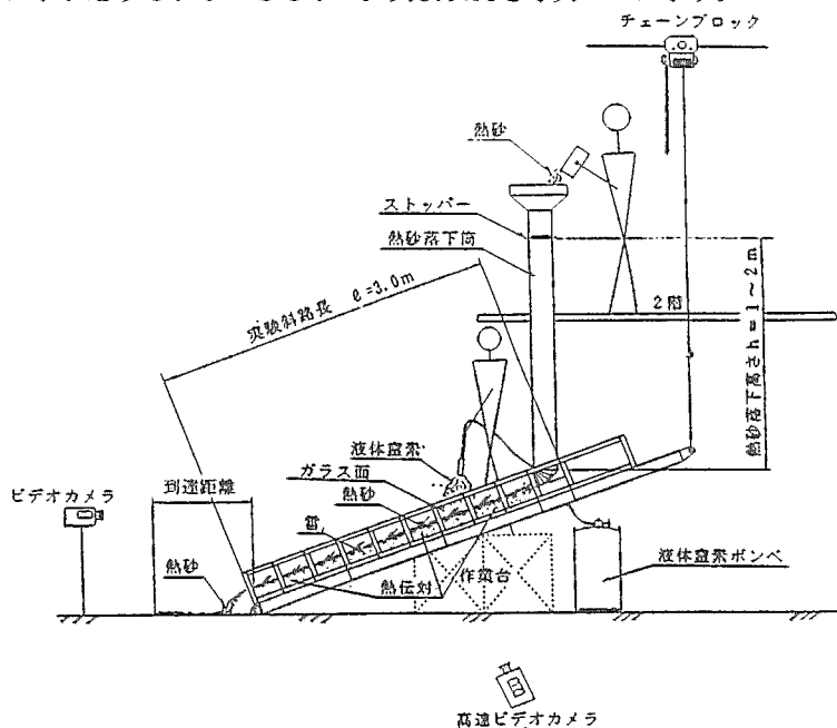
図-3 実験状態概念図
