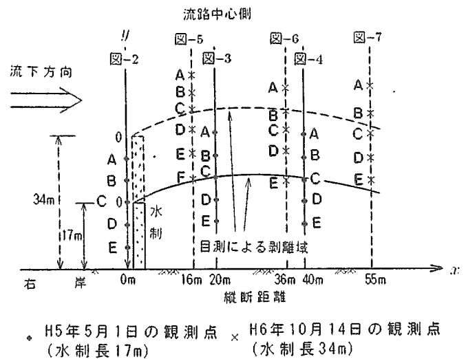
図-1 測定点平面図
