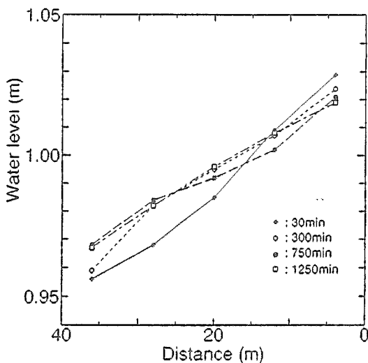
図-2 水面形の時間変化
