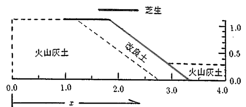
図-1 初期実験断面形状
