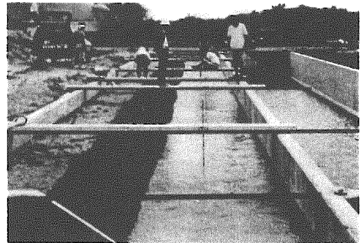
写真-1 芝河岸の浸食実験水路 (通水時)
