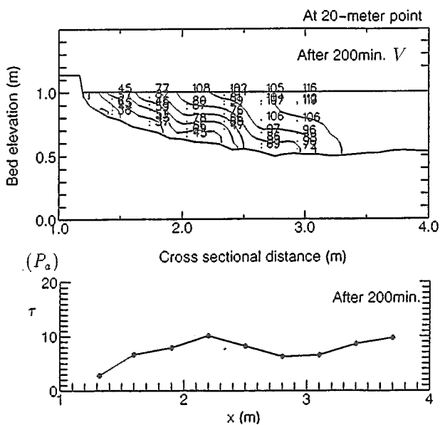
図-4 横断面、流速コンター、せん断力の時間変化
