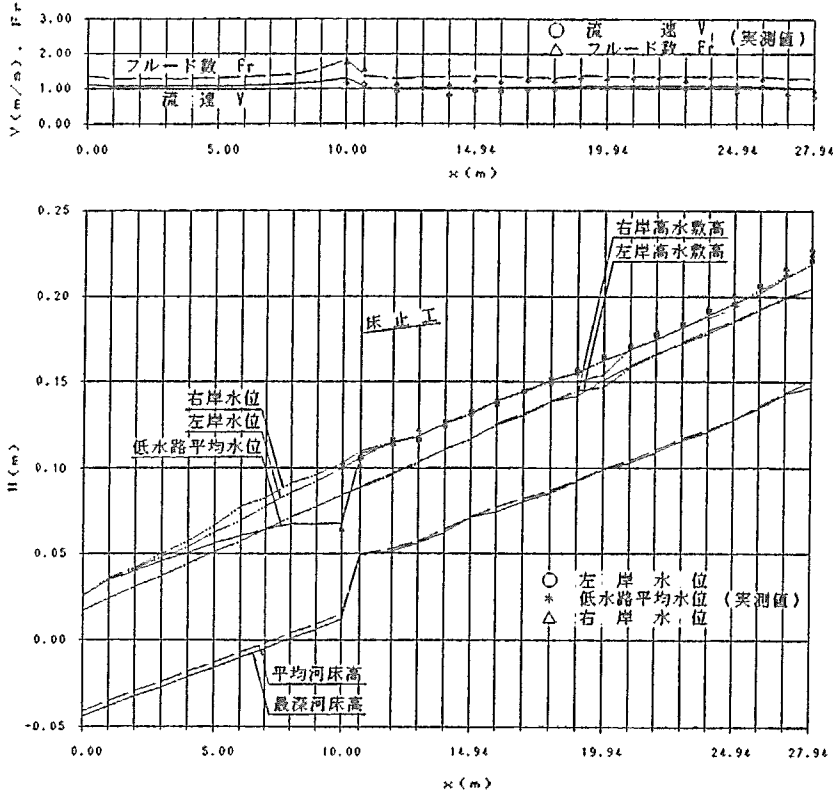
図-1 流速、フルード数、水位縦断面図
