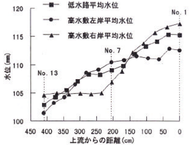
(a)実験結果(参考文献2)から引用)
