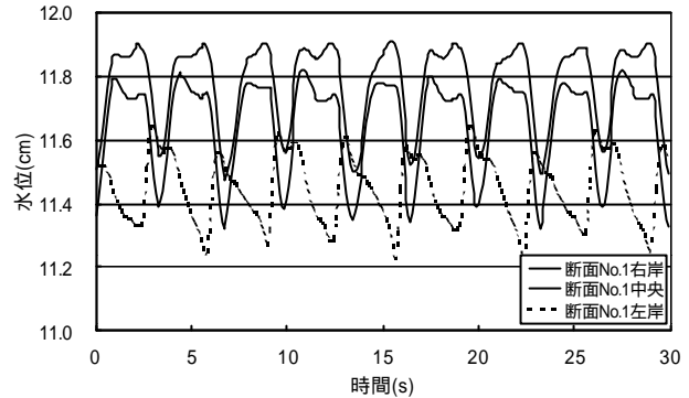
(b)本モデルによる計算
