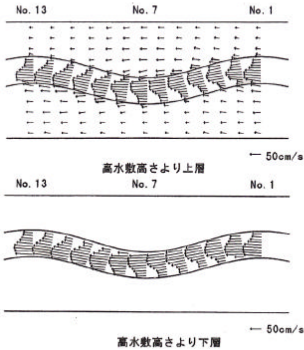
(a)実験結果(参考文献2)から引用)
