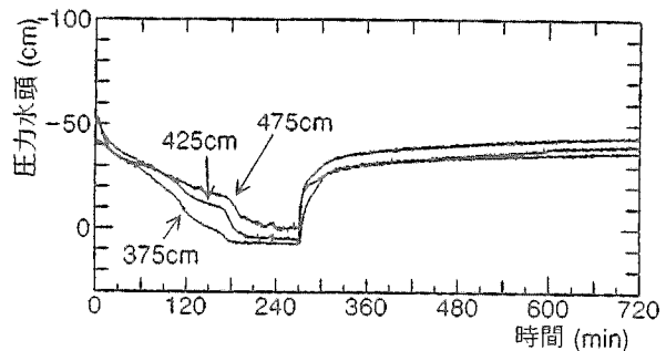
図3-3 表層付近の圧力水頭の変化 (下流側)
