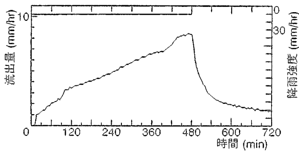
図3-5 CASE.2のR, Q
