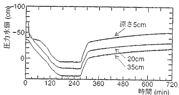
図3-4 375cm地点の圧力水頭の変化
