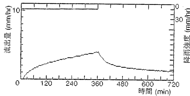
図3-6 CASE.3のR, Q
