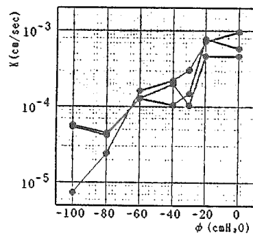
図2-3 圧力水頭 ( \phi ) と不飽和透水係数 ( k )
