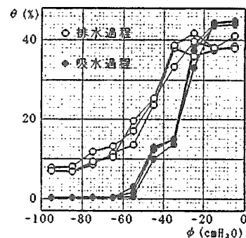
図2-2 圧力水頭 ( \phi ) と体積含水率 ( \theta )
