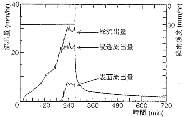
図3-1 CASE.1のR, Q
