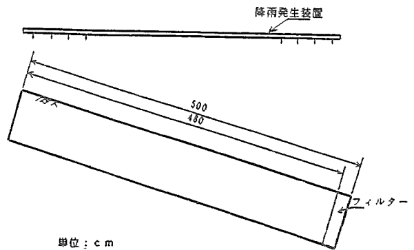
図2-1 実験装置の模式図
