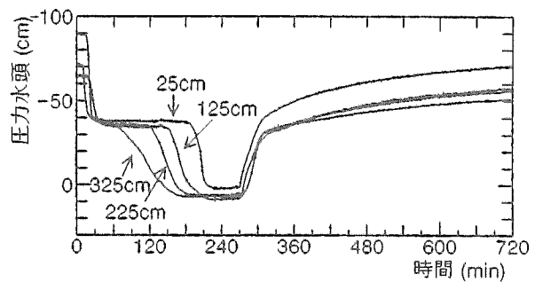
図3-2 表層付近の圧力水頭の変化 (上流側)
